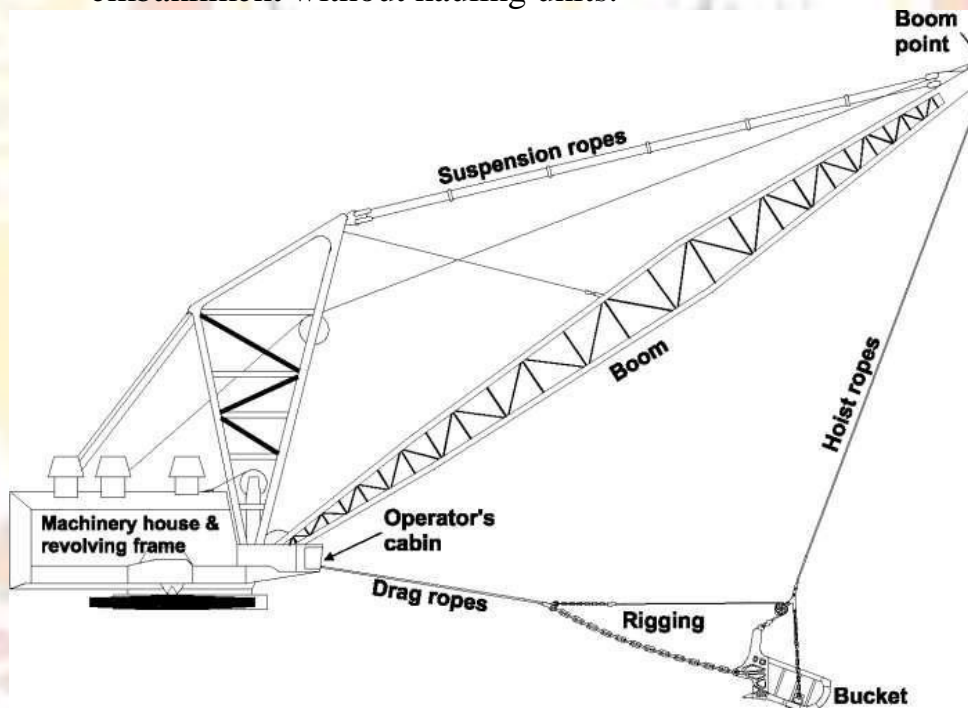
Fig. Dragline
