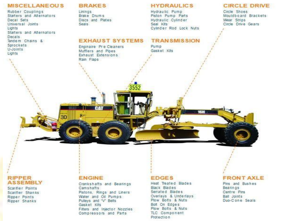
Fig. Grader
